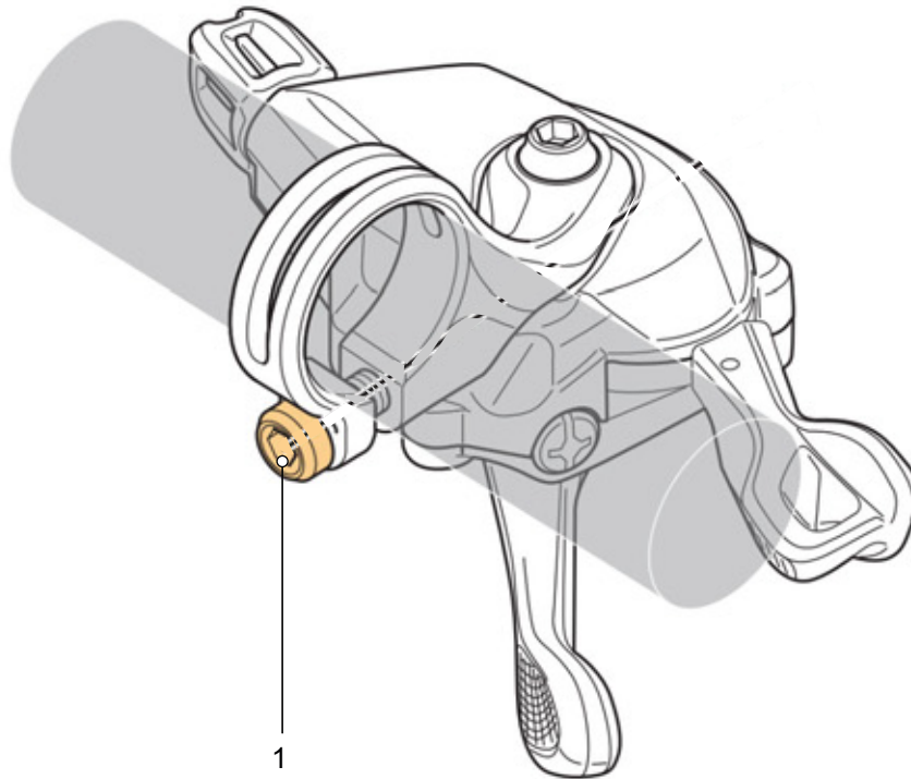
80 paveikslėlis. SHIMANO perjungimo svirties tvirtinimo varžto padėtis
