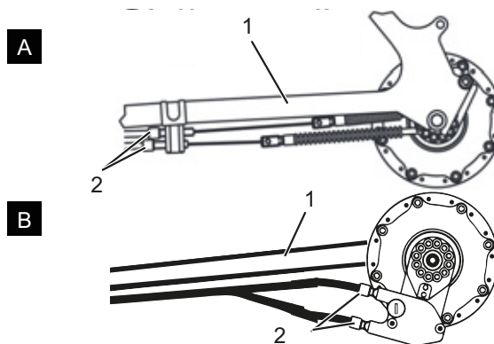
125 paveikslėlis. Dviejų pakopų, dviejų alternatyvių variantų (A ir B) reguliavimo įvorės (2), kabeliu valdoma pavarų perjungimo grandinės atrama (1)
