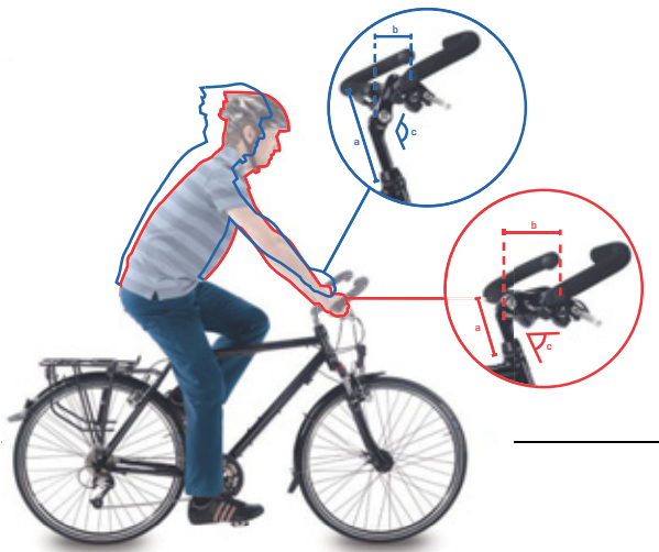
72 paveikslėlis. Miesto dviračio (mėlynas) ir turistinio dviračio (raudonas) padėtis
