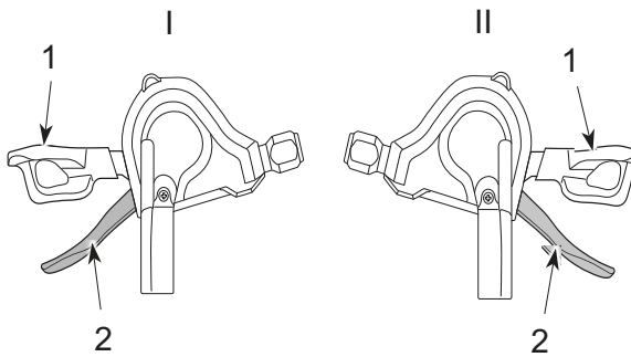
108 paveikslėlis. Kairiojo (I) ir dešiniojo (II) pavarų perjungimo mechanizmo perjungimo į žemesnę pavarą svirtis (1) ir perjungimo į aukštesnę pavarą svirtis (2)
