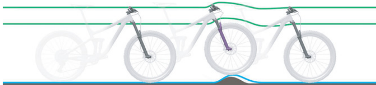
198 paveikslėlis. Per kietas amortizuojančių šakių slopinimas nelygumuose
